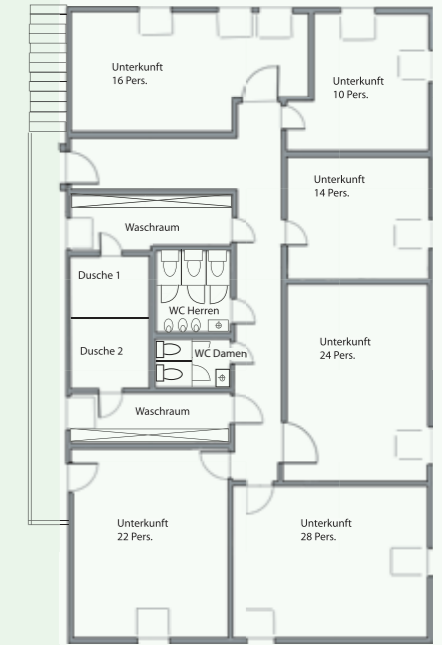
Obergeschoss
