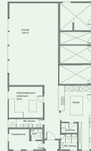
Erdgeschoss
